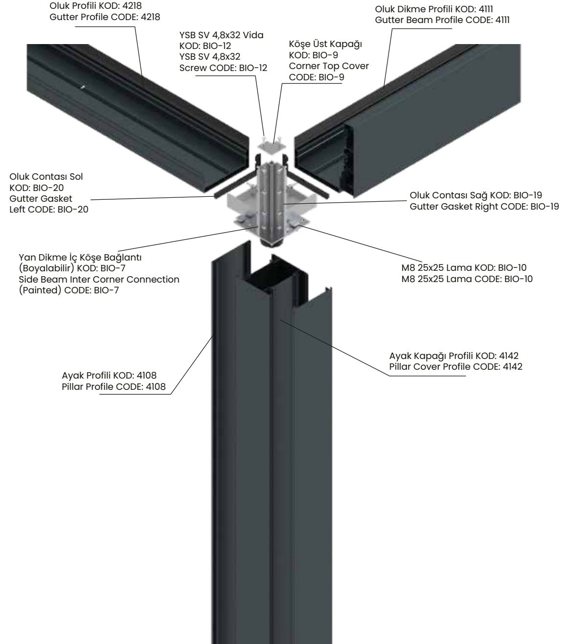
Ortak köşe aparatı-Common corner fitting
